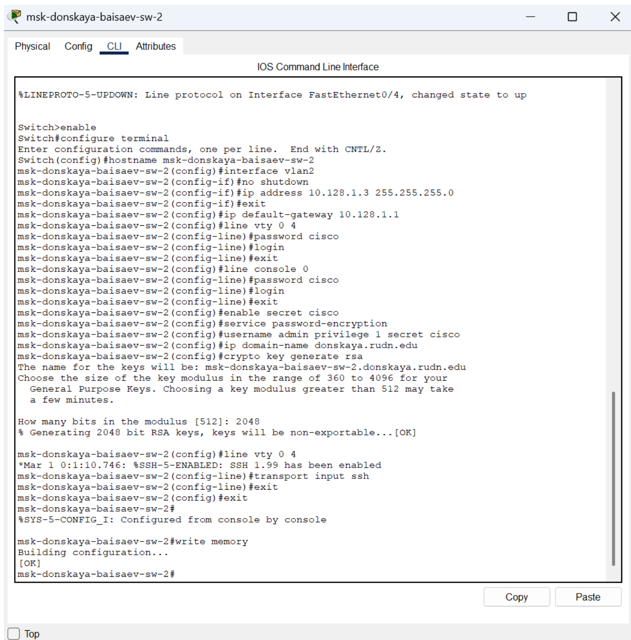
Рис. 1.4. Настройка коммутатора msk-donskaya-baisaev-sw-2, используя типовую конфигурацию.
