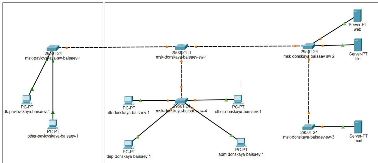
Рис. 1.2. Размещение коммутаторов и оконечных устройств согласно схеме сети L1.
