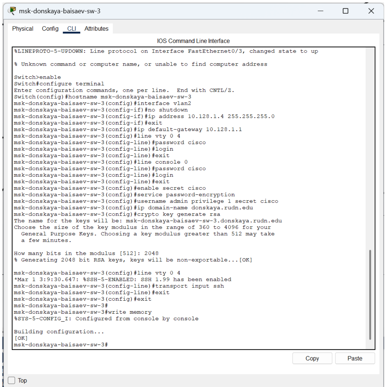
Рис. 1.5. Настройка коммутатора msk-donskaya-baisaev-sw-3, используя типовую конфигурацию.
