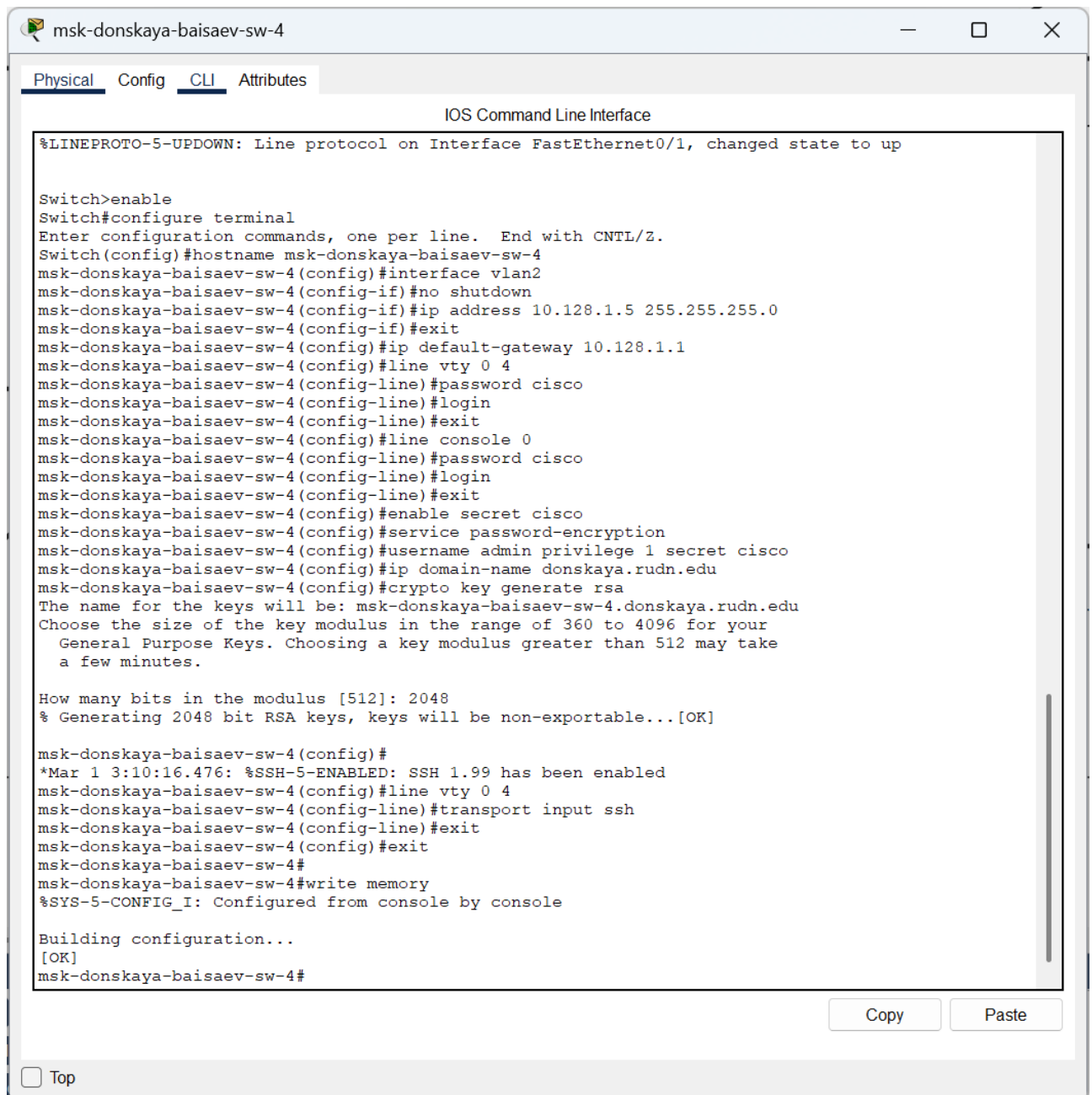
Рис. 1.6. Настройка коммутатора msk-donskaya-baisaev-sw-4, используя типовую конфигурацию.
